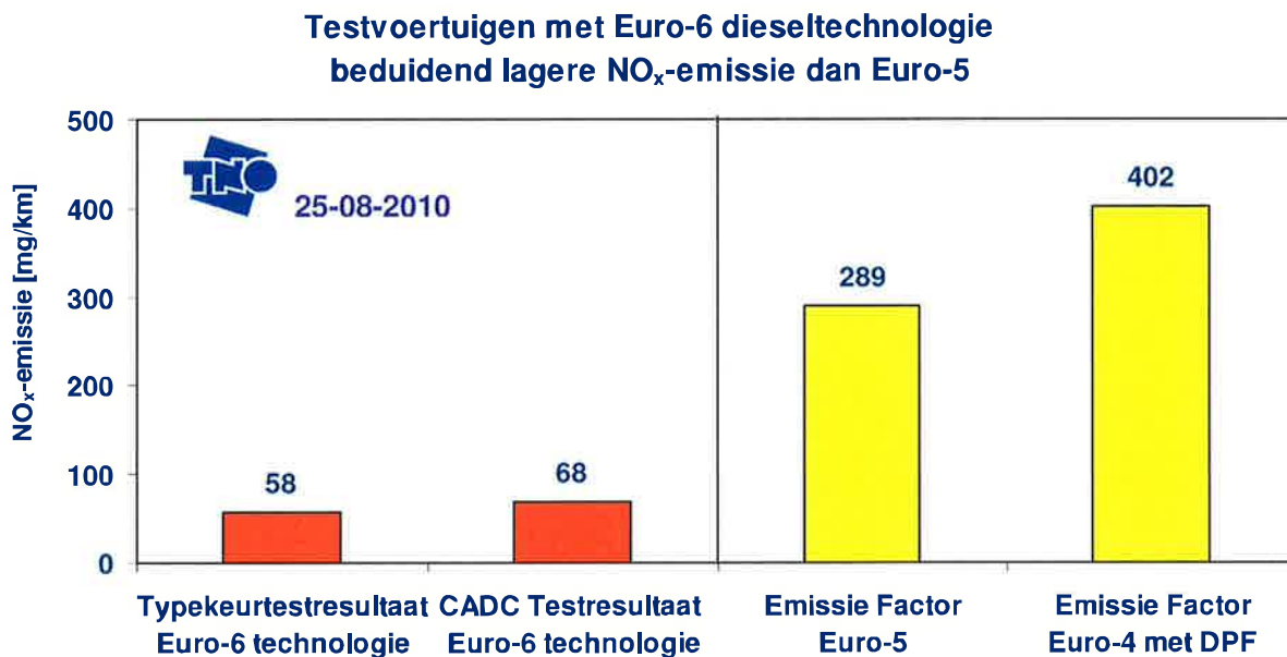
Figuur 9: gemiddelde NO x -emissie over praktijktestcyclus en de typekeurcyclus van de testvoertuigen met Euro-6 dieseltechnologie, ten opzichte van de CAR-emissiefactoren [4] voor Euro-5 en Euro-4 personenwagens met een dieselmotor en roetfilter (DPF)
