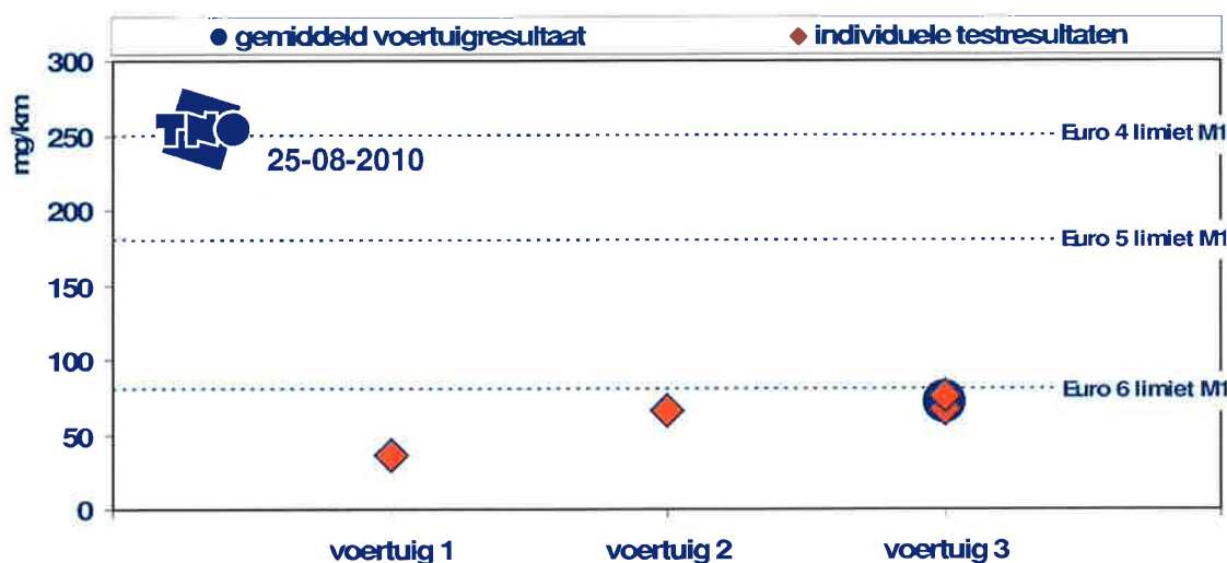
De testvoertuigen met Euro-6 technologie voldoen aan de voor Euro-6 gestelde diesel \text{NO}_x -limiet
