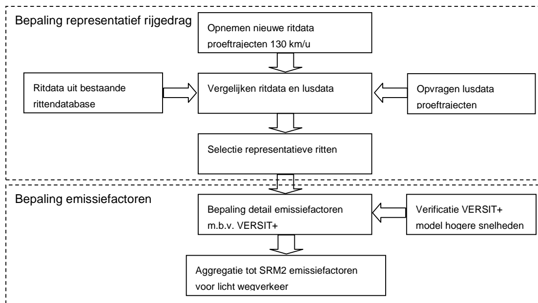
Figuur 1 Verschillende stappen voor het bepalen van emissiefactoren voor nieuwe verkeerssituaties
