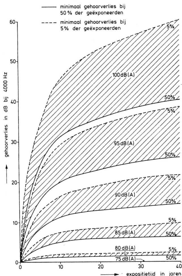
Grafiek 1 Geheerterverlies bij 4000 Hz als functie van de blootstellingsduur, voor geluidsniveaus op de arbeidsplaats van 75 tot 100 dB(A)
