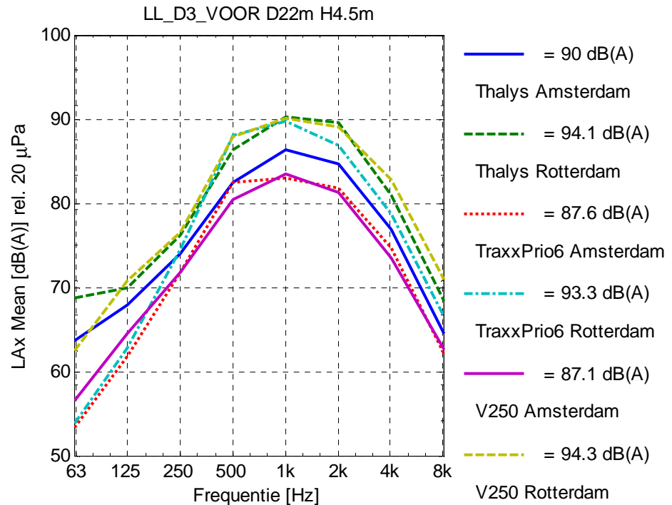
Figuur 17 Gemiddelde octaafspectra van het geluidexpositieniveau bij meetdoornede 3, Thalys, V250 en TraxxPrio in beide richtingen.
