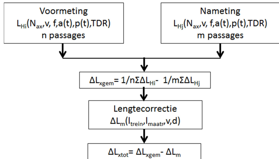
Figuur 10 Bepaling geluidreductie met uit verschillen in de overdracht L_H en lengte van de maatregel. N_{ax} = aantal assen, f = frequentie, a(t) = versnellingsignaal railtrilling, p(t) = geluidruksignaal, TDR = verticale afstandsdeмпing van de rail.
