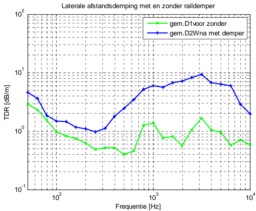
Figuur 83 Gemiddelde laterale afstandsdeмпing van D1 westspoor bij de voormeting en D2 westspoor met raildeмпers bij de nameting.
