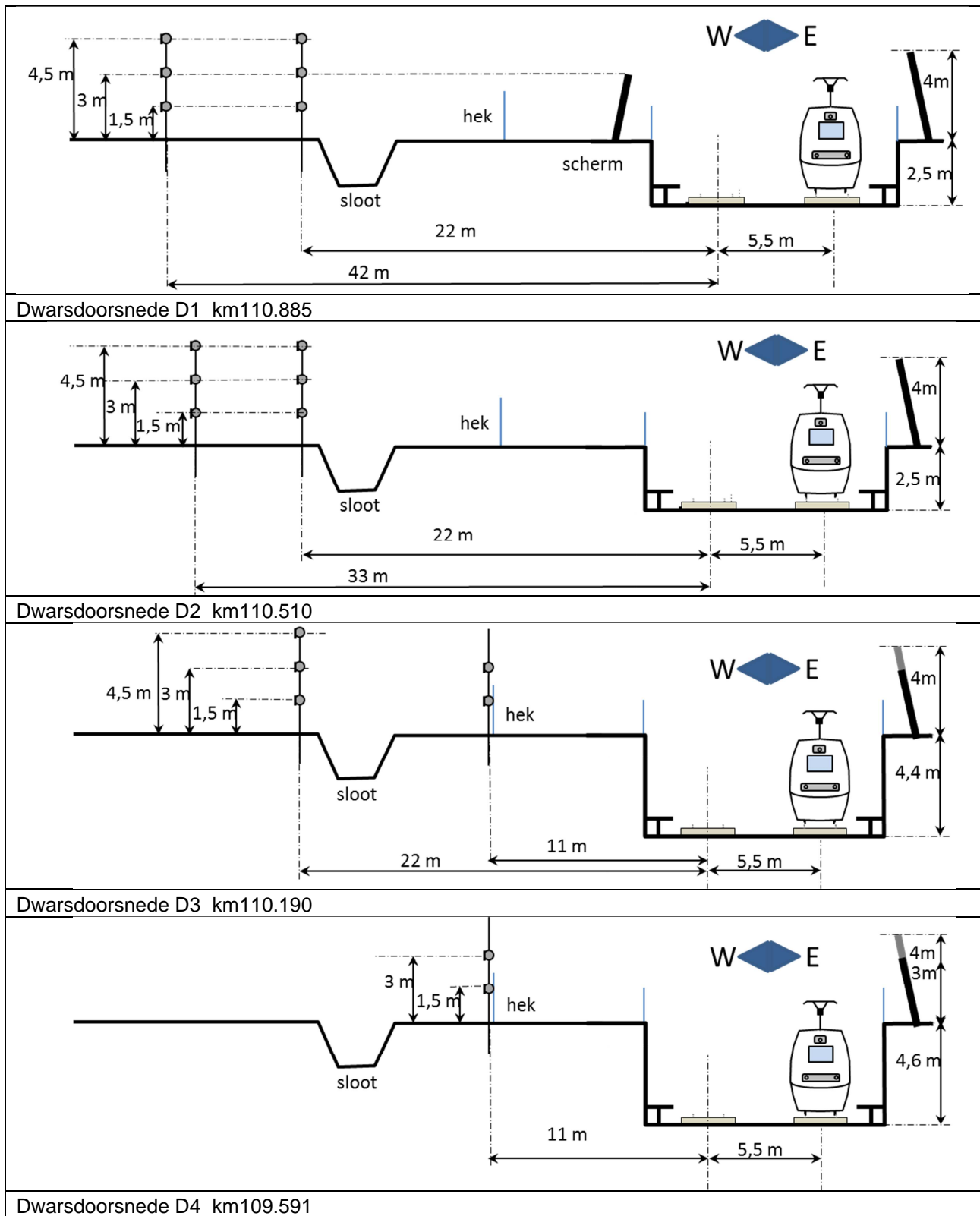
Figuur 5 Microfoonposities op meetdoorsnedes D1, D2, D3 en D4. Bij D3 en D4 is de schermhoogte 3 m, echter gaat deze na 10 m over in 4 m hoogte. De aanzicht van de doorsnede is gericht naar Amsterdam, met de westkant links.
