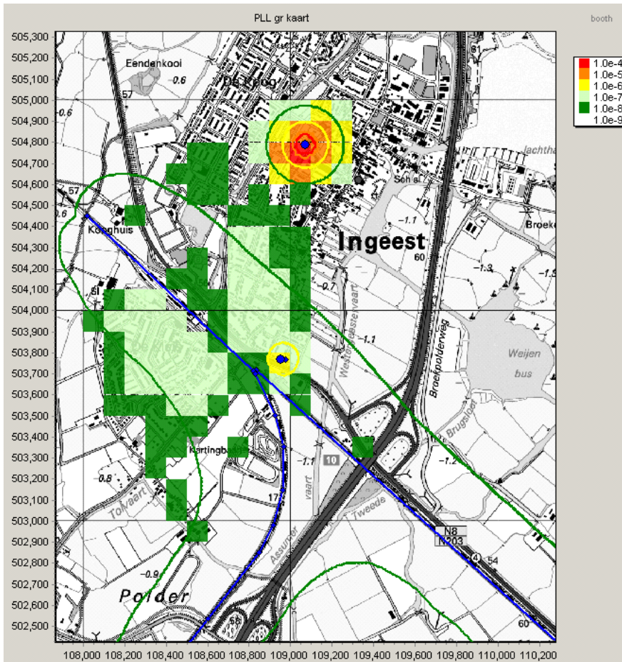
Figuur 2-2 PLL GR -kaart met plaatsgebonden risicocontouren
