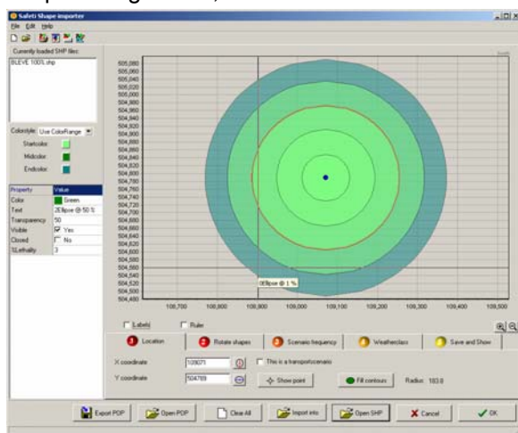
Figuur B-1 BLEVE met de 90%, 50% 10% en 1% letaliteitscirkels
