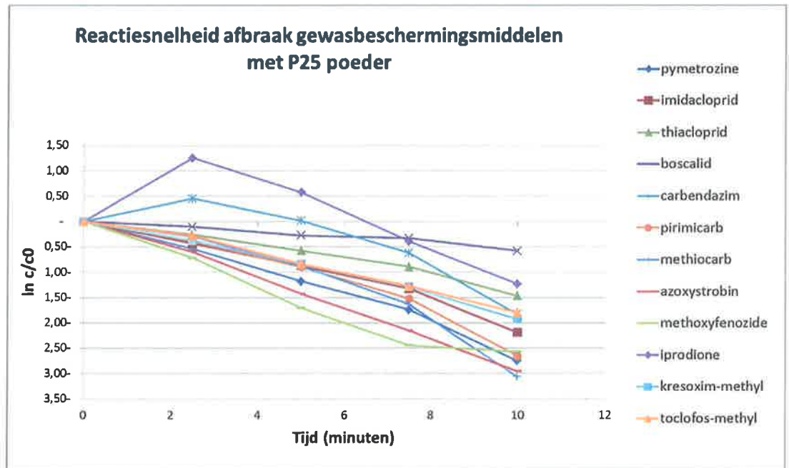
Figuur 31: Afbraak gewasbeschermingsmiddelen (startconcentratie 50-780 ng/ml per middel; 10 W/m 2 UV-A)
