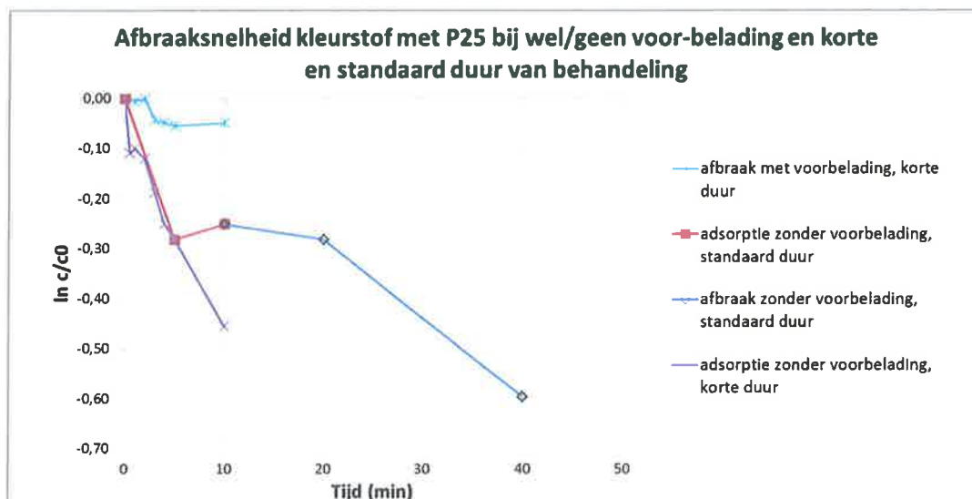
Figuur 18: Afbraaksnelheid voor P25 en effect van wel/geen voorbelading
