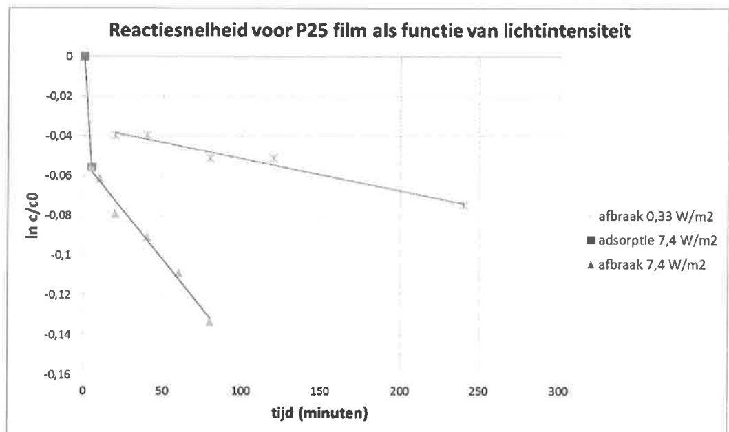
Figuur 30: Effect lichtintensiteit op afbraaksnelheid Reactive Blue door P25 film
