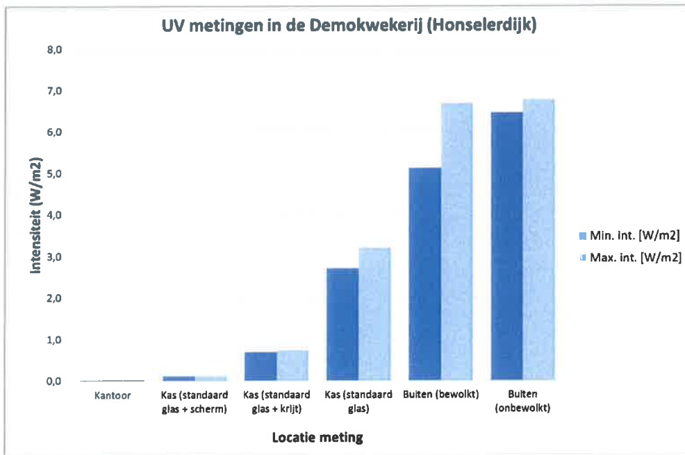
Figuur 3: UV-A beschikbaarheid in de kas (gemeten op 28 augustus 2012, rond 12:00; wisselvallige dag)
