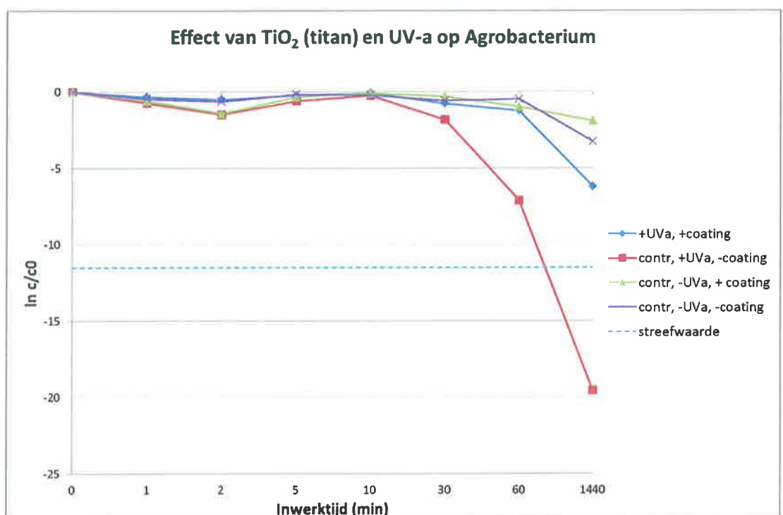
Figuur 34: Afbraak Agrobacterium Rhizogenes in de tijd met FKO (intensiteit ca 15 W/m 2 , initieel hoeveelheid bacteriën 3,7 \cdot 10^{10} CFU)
