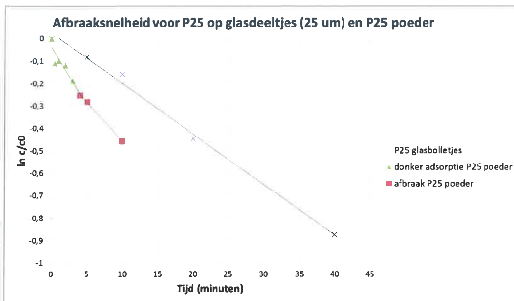
Figuur 19: Afbraaksnelheid Reactive Blue voor glaspereis met P25 coating
