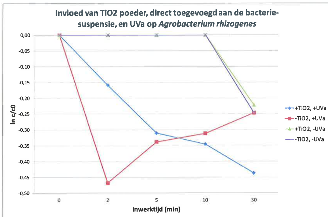
Figuur 37: Resultaten desinfectieproef met P25 poeder in petrischaal (15 W/m 2 ; starthoeveelheid bacteriën = 4,9 \cdot 10^9 CFU)
