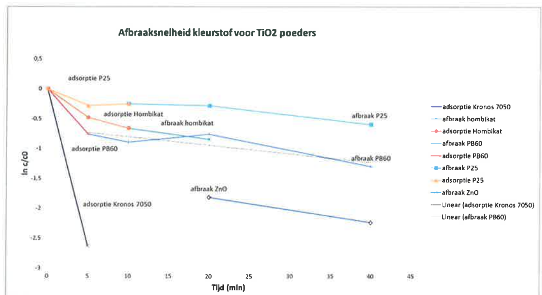
Figuur 17: Afbraaksnelheid Reactive Blue voor de TiO 2 poeders (lijnen zijn ter illustratie ; voor ZnO en Kronos 7050 konden respectievelijk geen goed adsorptie/afbraak verloop bepaald worden)
