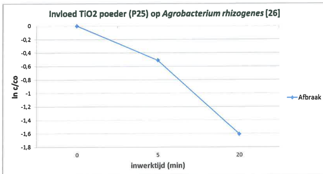
Figuur 38: Resultaten desinfectieproeven met P25 poeder door Amenedi et al. [26] ( 6,4 \text{ W/m}^2 , starthoeveelheid bacteriën = 3,6 \cdot 10^7 )
