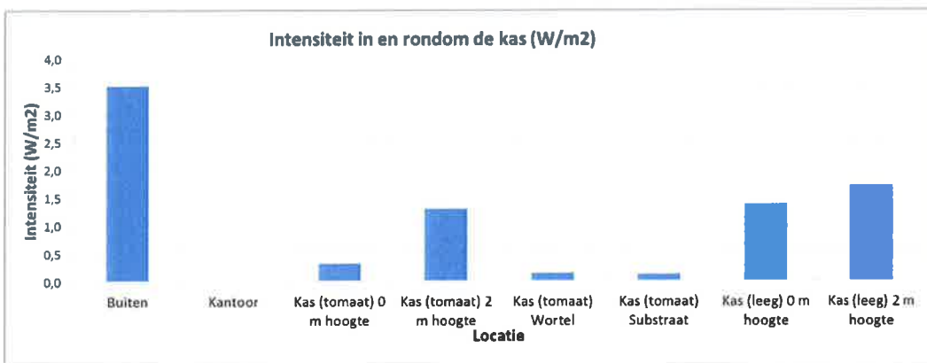
Figuur 4: UV-A beschikbaarheid in de kas (gemeten op 26 oktober 2012, bewolkte dag)
