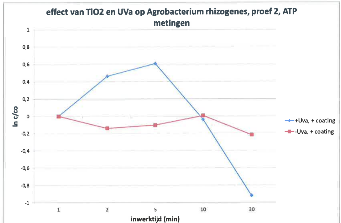
Figuur 35: Resultaten afdoding Agrobacterium in recirculatie-opstelling (ATP metingen; 7 W/m 2 ; starthoeveelheid bacteriën = 2,44*10 11 CFU)
