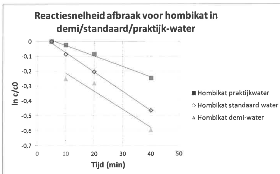
Figuur 25: afbraaksnelheid Reactive Blue in demi-, standaard- of praktijkwater voor Hombikat poeder
