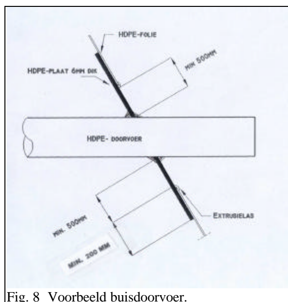
Fig. 8 Voorbeeld buisdoorvoer.
