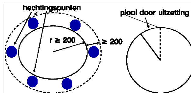
Fig. 16 Uitvoering (maatvoering en hechting) van een reparatiefolie
