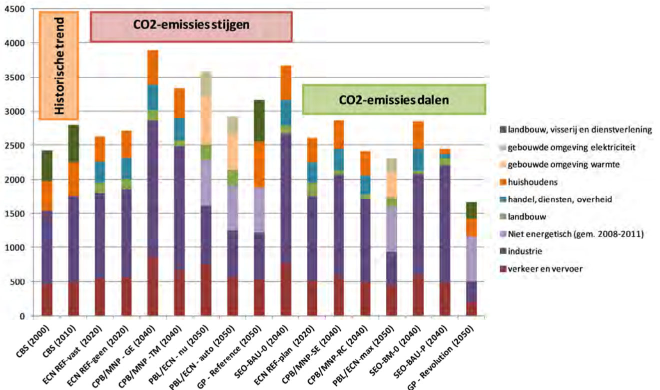
Figuur 3.6 Energievraag per sector (PJ) in Nederlandse toekomstscenario's. Indien een studie de niet-energetische energievrage in de industrie buiten beschouwing heeft gelaten, is ter referentie het gemiddelde van de niet-energetische energievrage in de jaren 2008-2011 toegevoegd.
