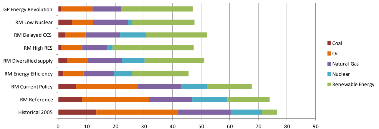
Figuur 3.1: Europees primair energieaanbod in 2050 (in EJ). RM: Roadmap scenario's van EC, GP: GreenPeace.
